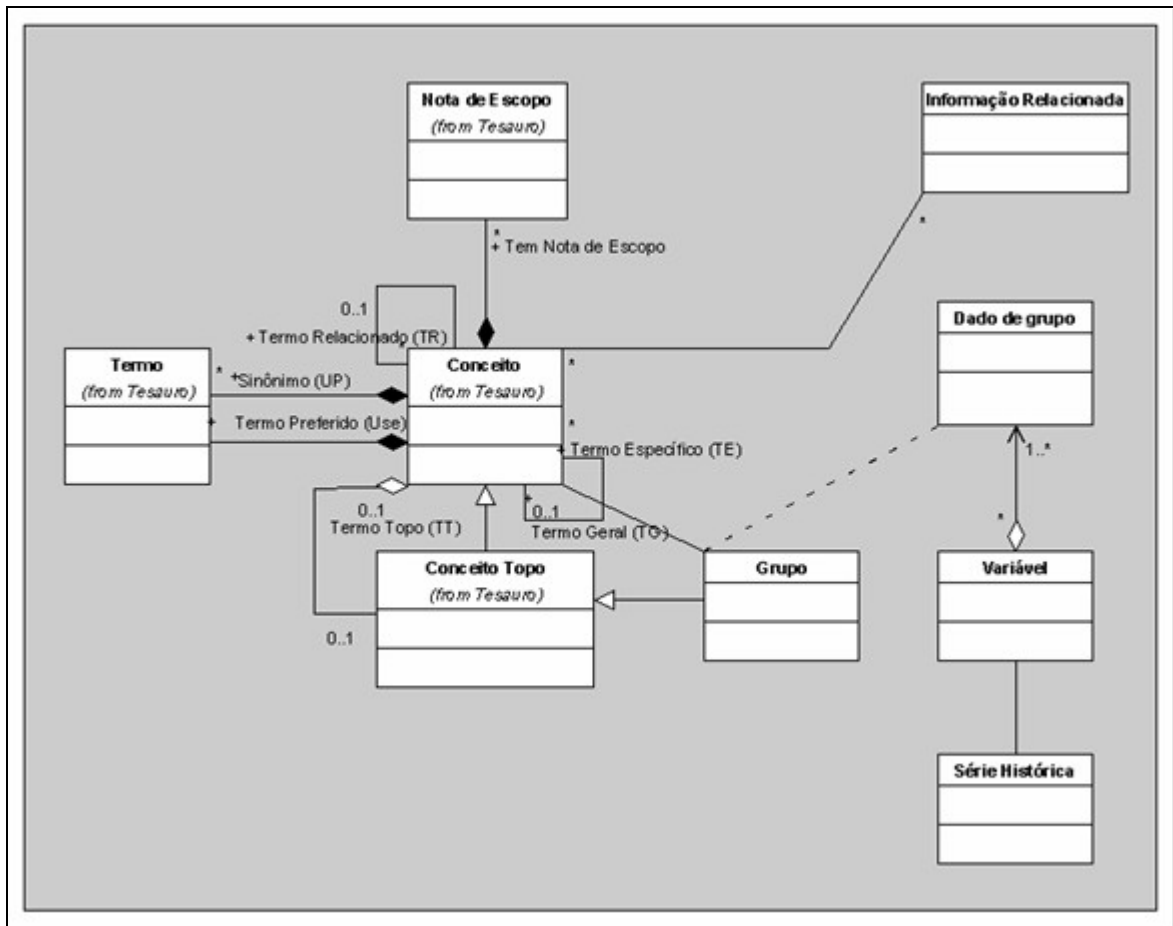
Diagrama 4 - Diagrama de Classes de SERVE
