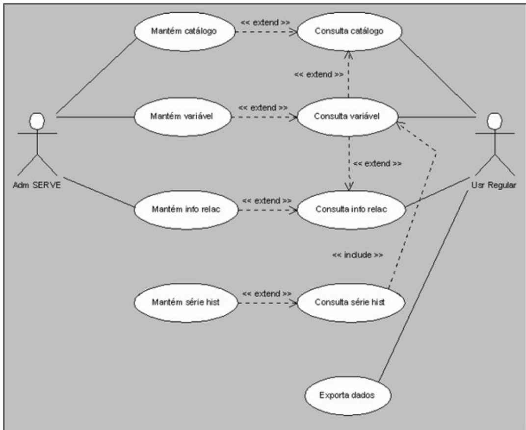
Diagrama 3 - Diagrama de Casos de Uso de SERVE
