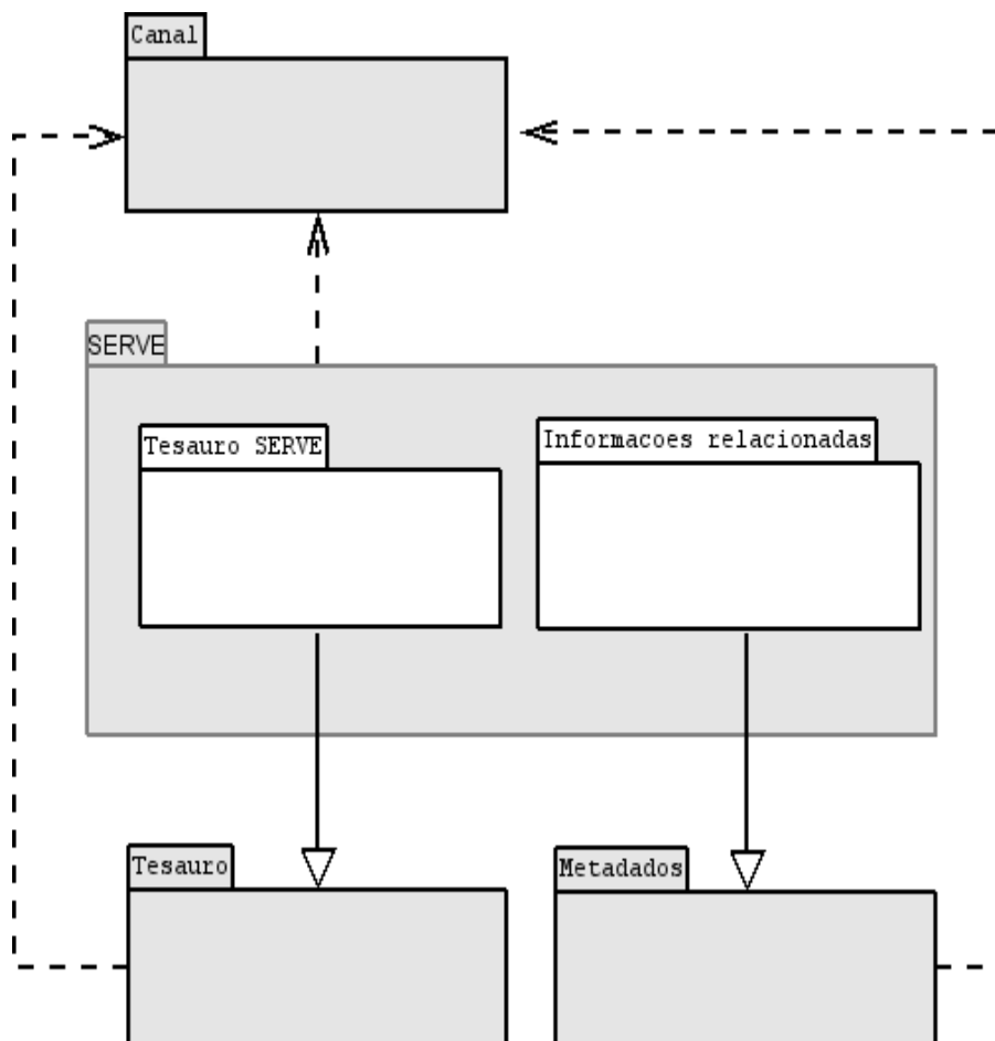
Diagrama 1 - Diagrama de Domínios
